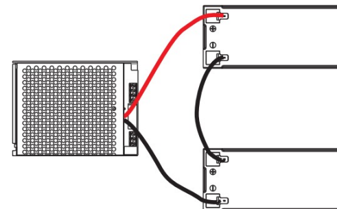
Рисунок 2. Схема подключения 2-х АКБ 12 В.
